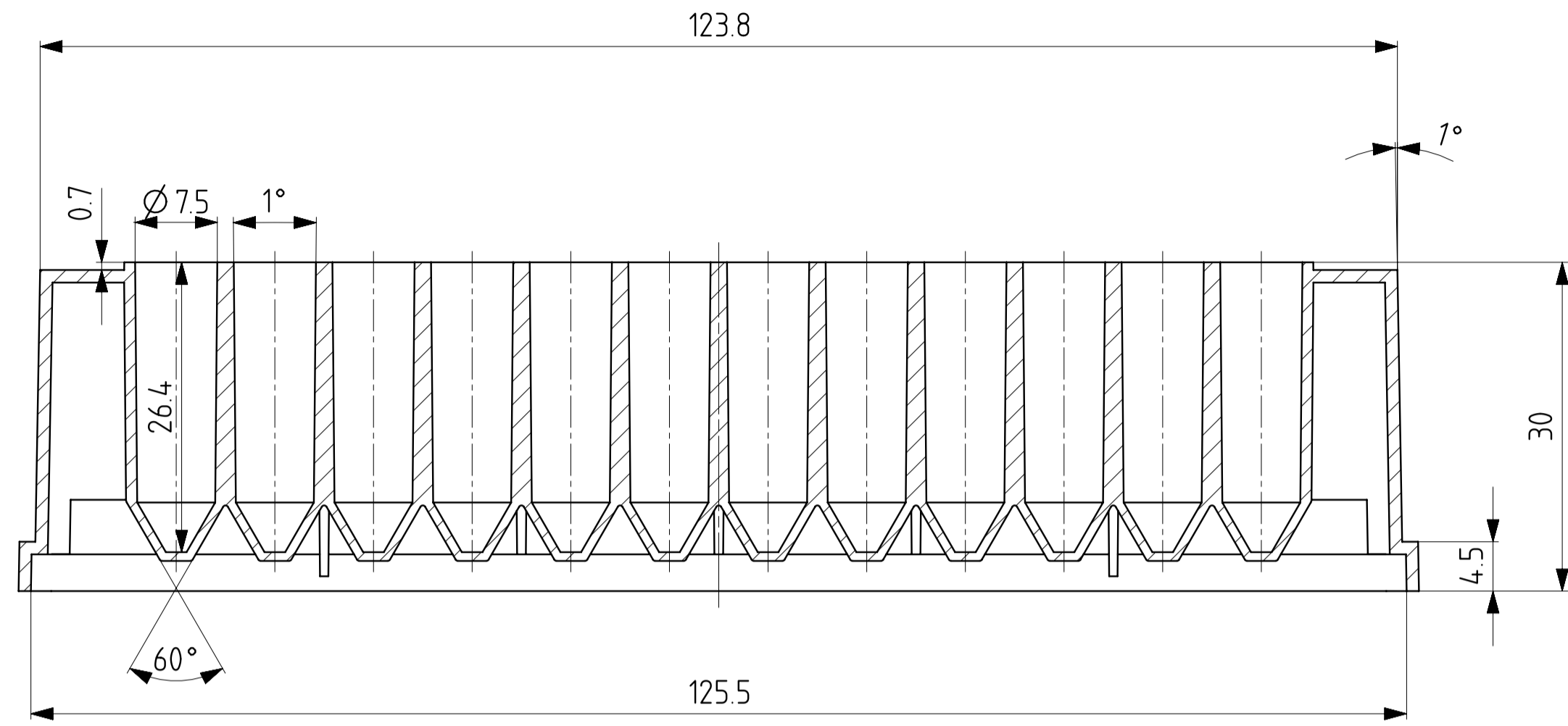
SECTION A-A
